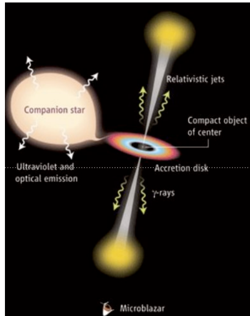
Figure 1 : «Vue d'artiste d'un astre compact dans un système binaire mettant en évidence les différentes composantes d'émission. La matière aspirée par l'objet compact s'enroule en un disque d'accrétion et se retrouve éjectée par l'intermédiaire des jets relativistes, à l'origine d'un intense rayonnement radio.»
