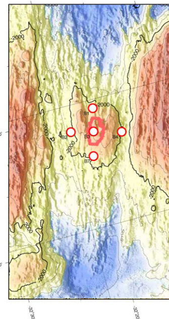
Image bathymétrique du volcan sous-marin Lucky Strike. Les stations sismologiques sont indiquées par des cercles et les contours de la chambre magmatique par le trait rouge. Le site hydrothermal se coïncide avec le cercle centrale.
